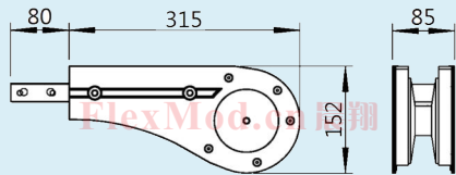
CXBEJ A85 Idler end unit (从动单元)
